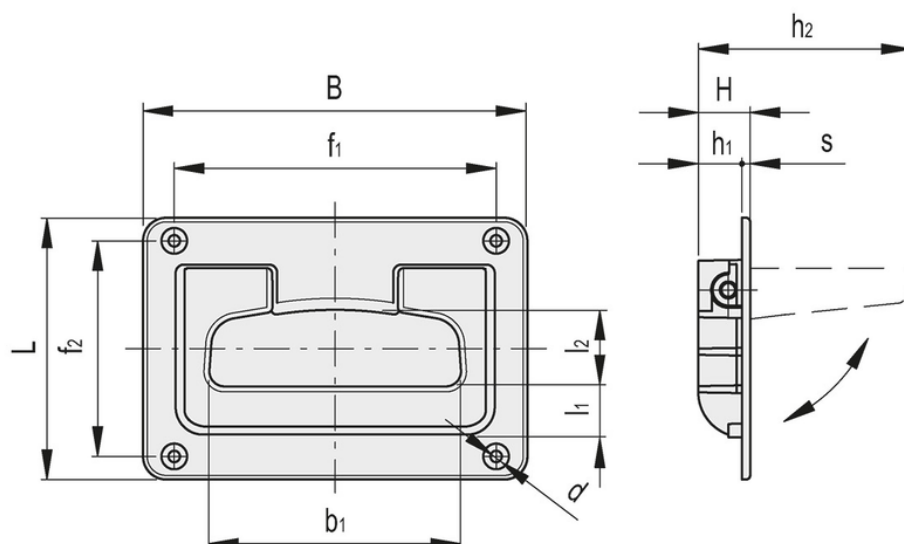
Rys.2: Budowa oraz zasada działania uchwytu MPR
