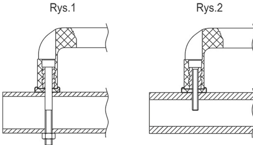
Rys. B: Sposoby montażu uchwytu M.643-FM za pomocą adaptera ADT na profilu okrągłym
