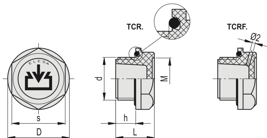
Rys.1. Budowa korka wlewowego TCR; TCRF
