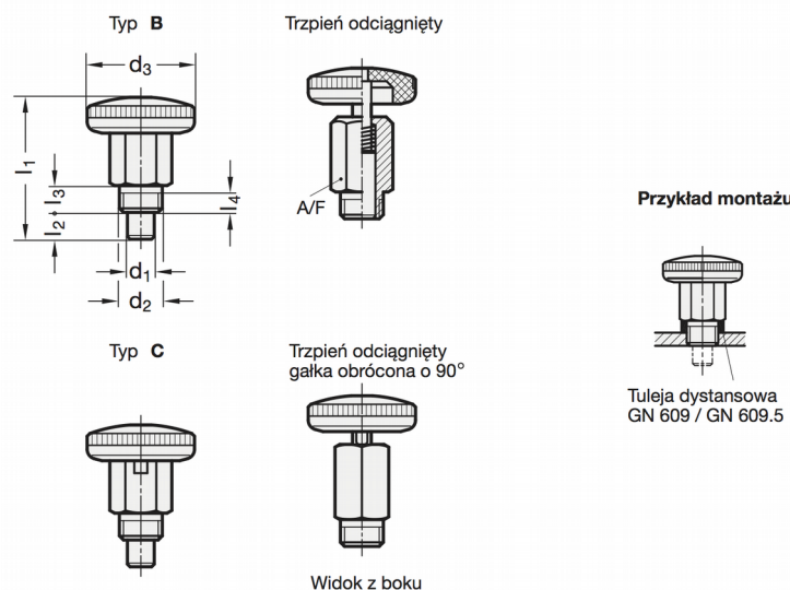
Rys.2 Konstrukcja trzpieni GN 822-RT i GN 822.1-RT.
