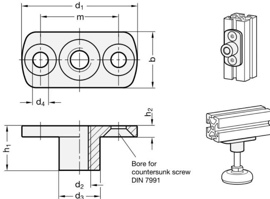
Rys.2. Budowa oraz przykład montażu GN 3490
