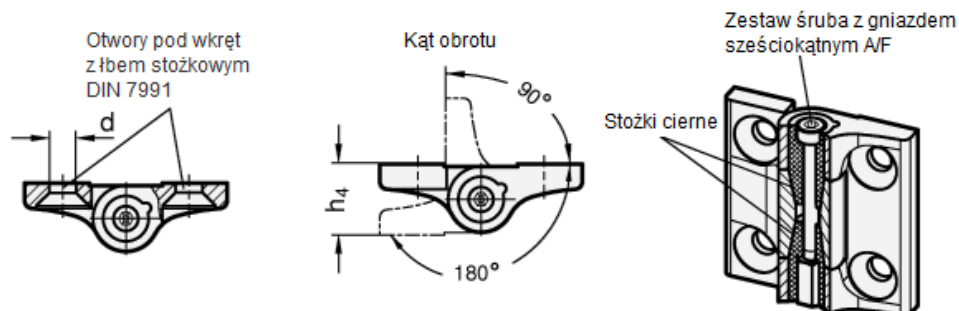
Rys. 2. Budowa zawiasu GN 437
