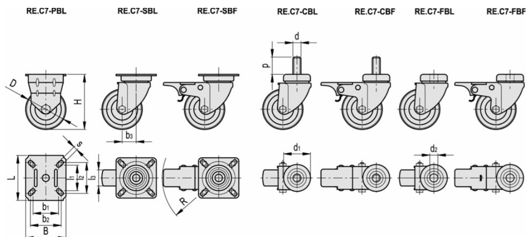
Rys.3. Zestawy kołowe RE.C7- możliwe wykonania standardowe
