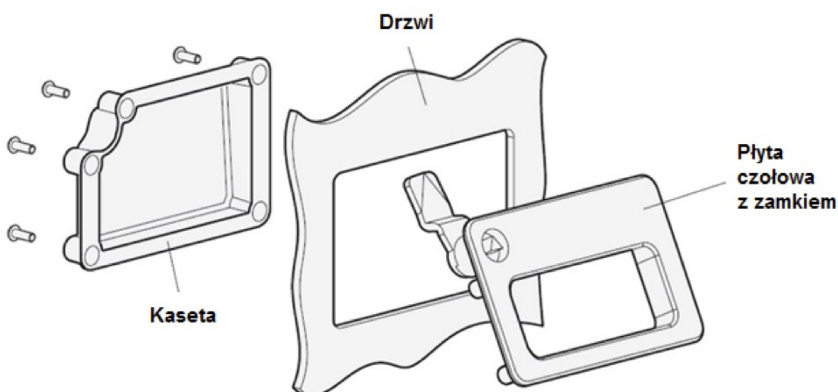
Rys.2. Budowa uchwytu kasetowego z zamkiem GN 115.10
