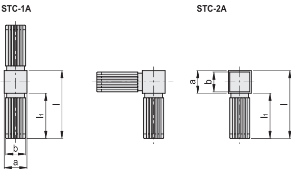
Rysunek pokazuje zmontowany łącznik. Dwie połówki łącznika z technopolimeru mogą mieć różne kształty lub wymiary zależnie od wariantu łącznika.
