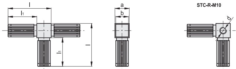
Rysunek pokazuje zmontowany łącznik. Dwie połówki łącznika z technopolimeru mogą mieć różne kształty lub wymiary zależnie od wariantu łącznika.
