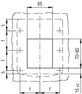
Schemat otworów
