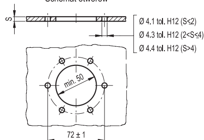
Schemat otworów
