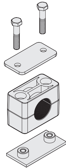
DCK-S-*-SRE-PU-PL (*Grupa 2÷7)
