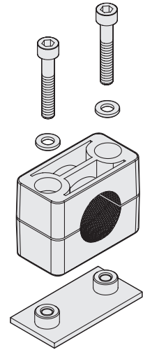
DCK-S-*-SRC-WA-PL (*Grupa 2÷7)
