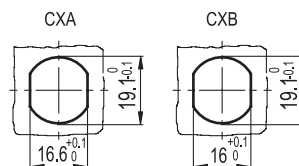
Otworki montażowe
