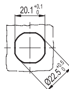
Otwór montażowy
