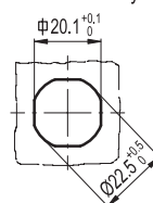
Otwór montażowy
