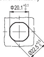
Otwór montażowy
