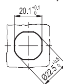
Otwór montażowy
