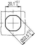
Otwór montażowy
